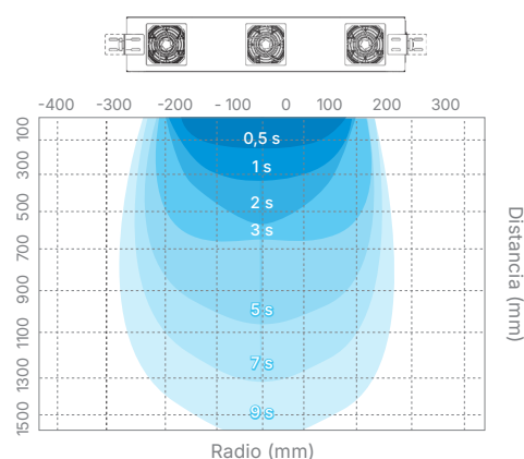
Imagen 2. Tiempo de decaimiento (en segundos) en el FU432S
